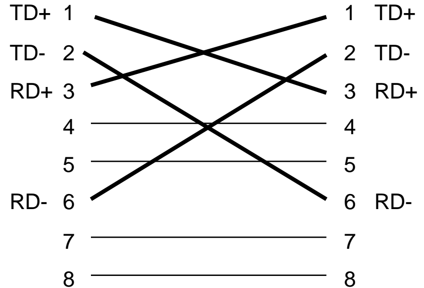
Połączenie krosowe
