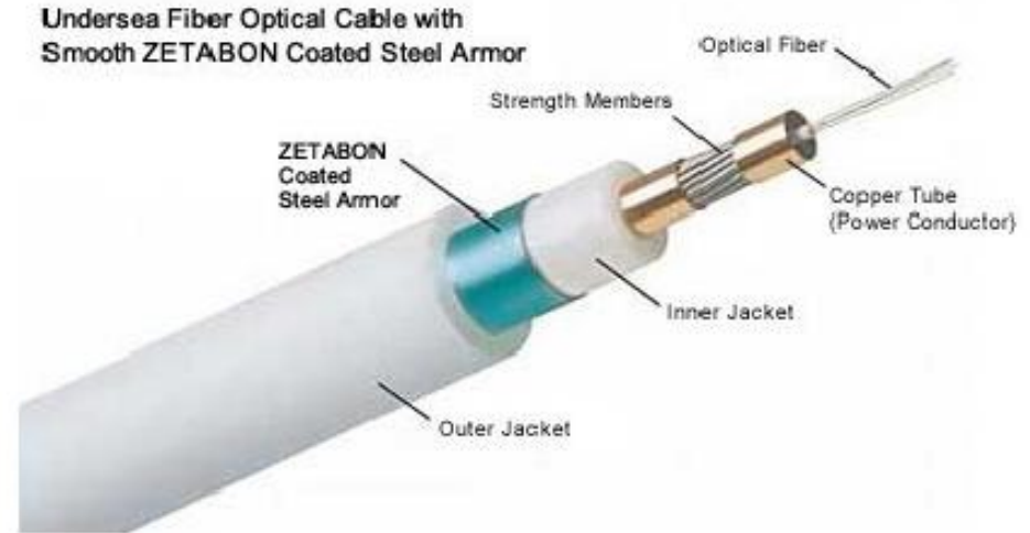
Fiber 1980 (30'000-300'000 Voice-Ch.)
